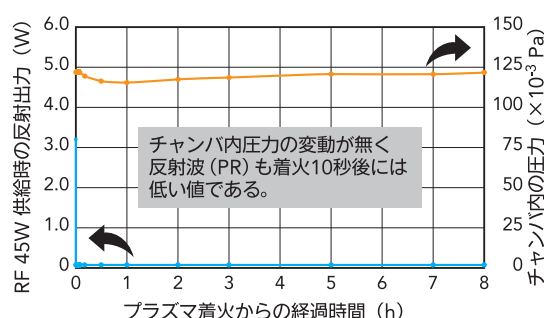
図 プラズマ安定性に関する検討結果 (プラズマ着火からのチャンバ内圧力と反射波の推移)
