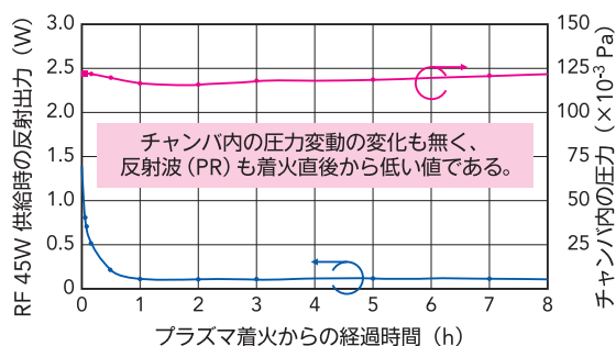
図 プラズマ安定性に関する検討結果 （プラズマ着火からのチャンバ内圧力と反射波の推移）
